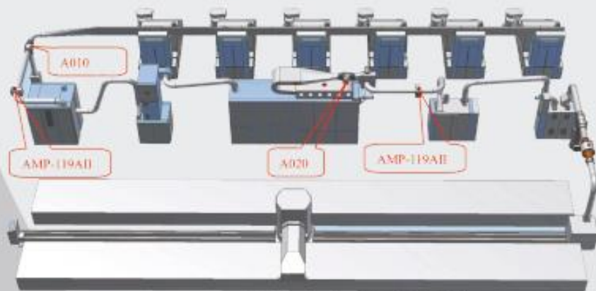
AMP-119AII 型火花探除器在清梳联上的安装
